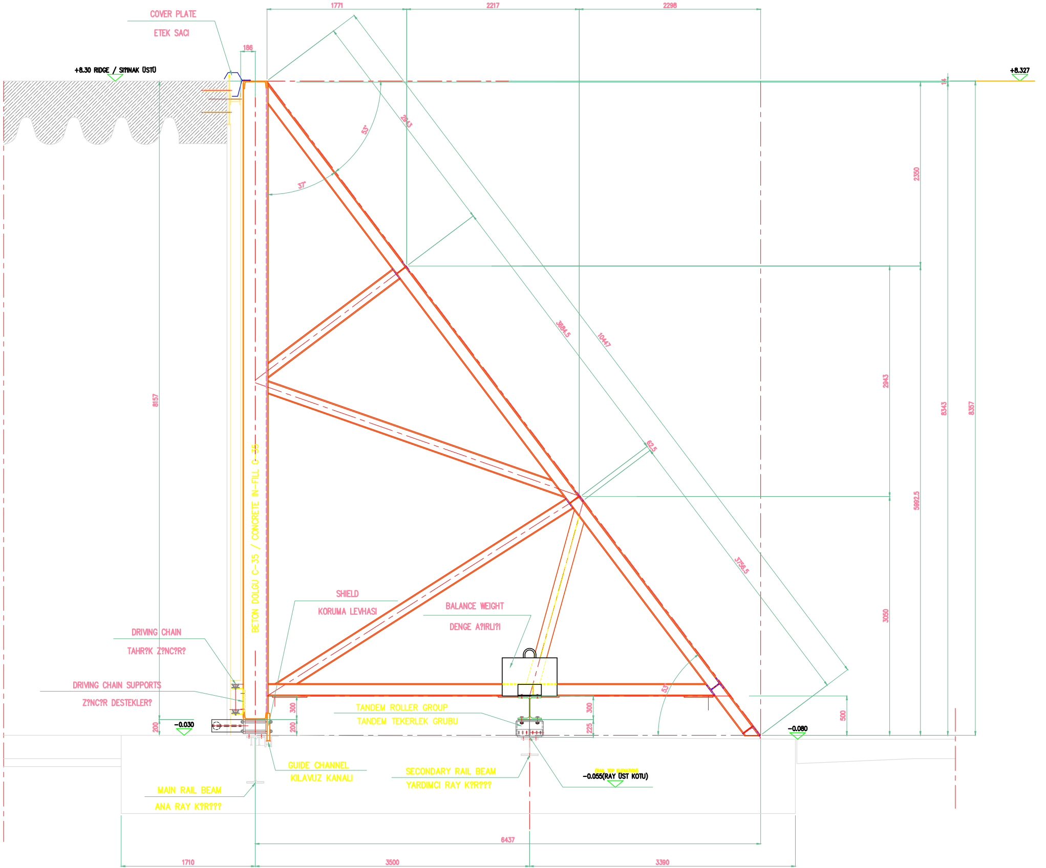
SECTION A-A Scale/Ölçek: 1/25 KESİT A-A
